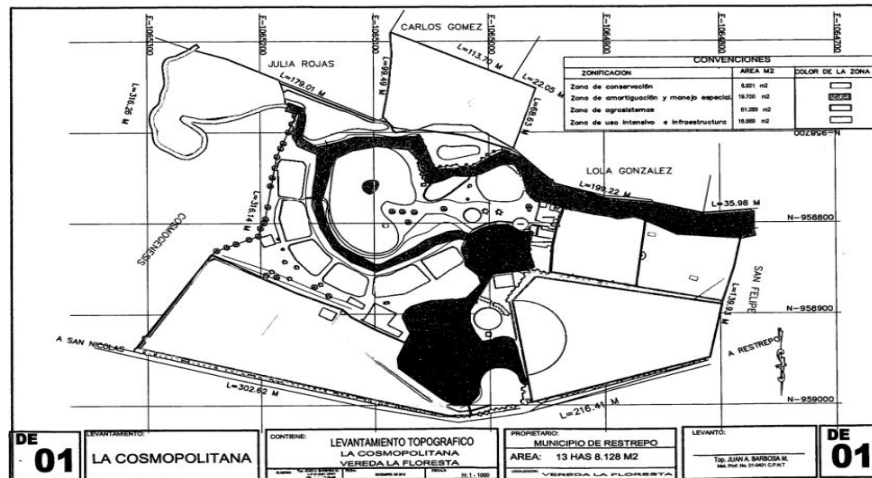
Figura 3. Levantamiento topográfico de la RNSC "LA COSMOPOLITANA" remitido en el marco de la solicitud de registro.
