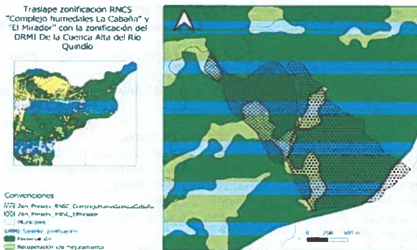
Figura 2. Zonificación RNSC Complejo De Humedales La Cabaña Y El Mirador y zonificación DRMI.
