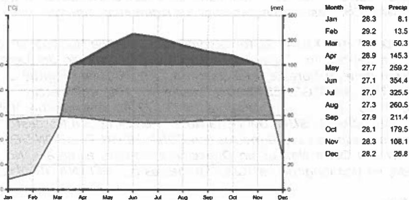
Temperature Mean: 28.1 °C Precipitation Sum: 1942.7 mm Figura 1 Diagrama ombrotérmico sitio "FI CUNAVICHE". Fuente: Climatecharts, 2024
