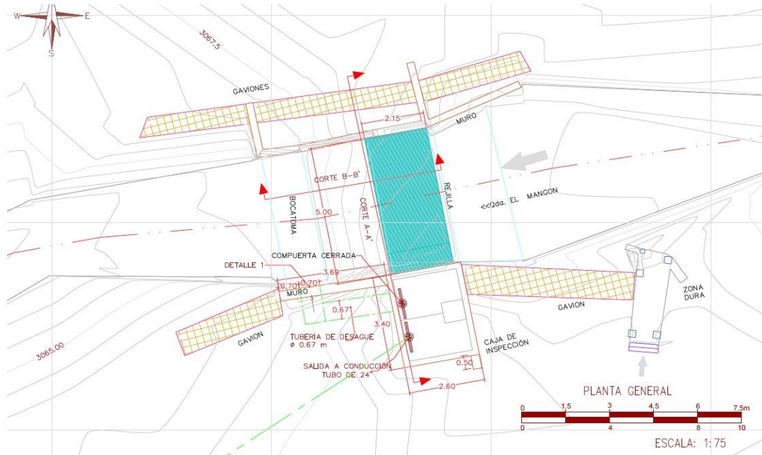
Imagen 1. Esquema de la captación
