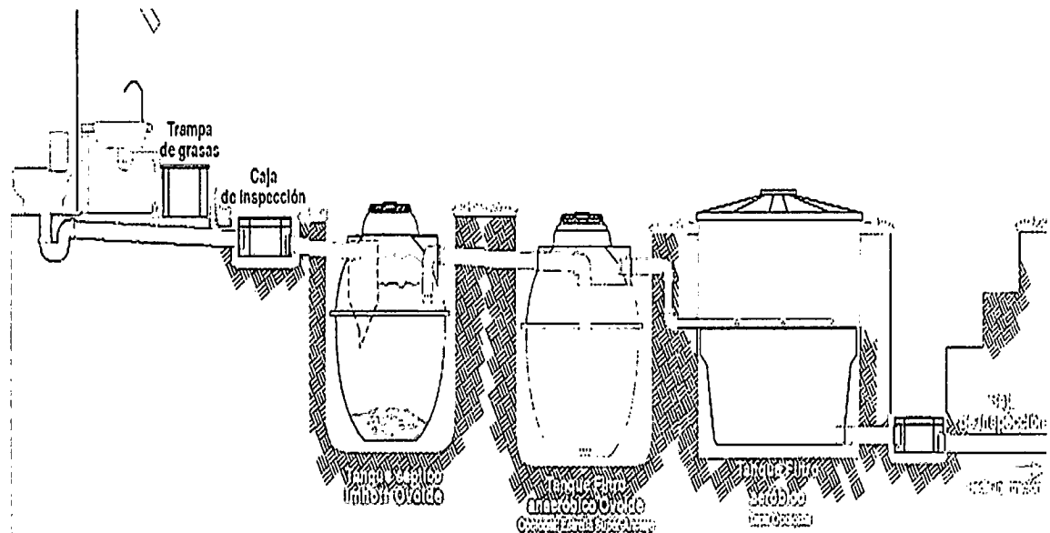
Imagen 2. Esquema general del STARD. (Fuente: EAB_ESP)
